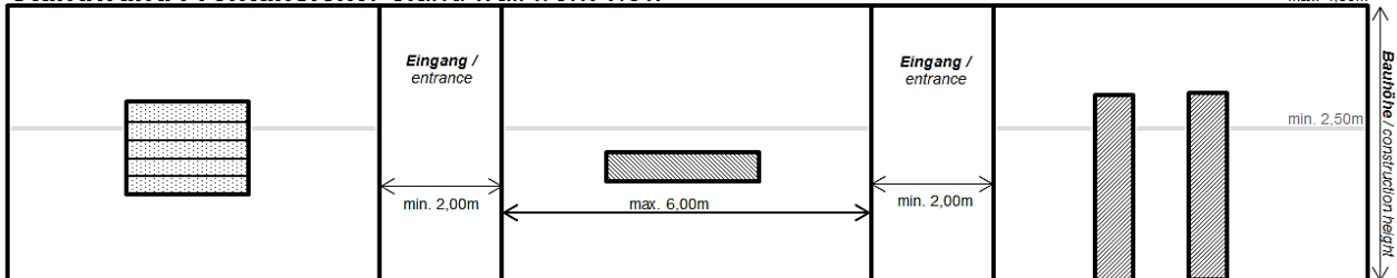
Standwand Frontansicht / stand wall front view
